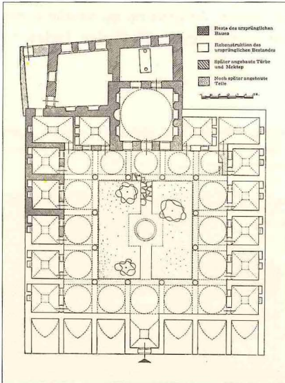
Ebülfazl Mahmud Efendi Medresesi'nin restitüsyon planı (Eyice, TD , sy. 14 [1959], s. 159)
