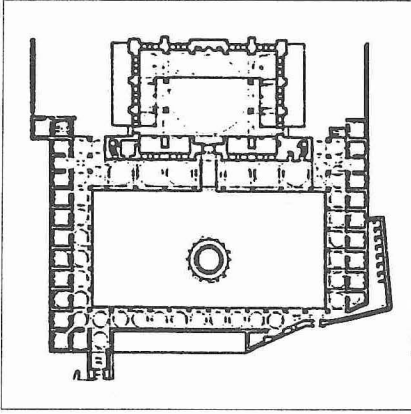
Edirnekapı Camii ve Medresesi'nin planı
