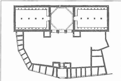
Ekmekcizâde Ahmed Paşa Kervansarayı ve planı - Edirne
