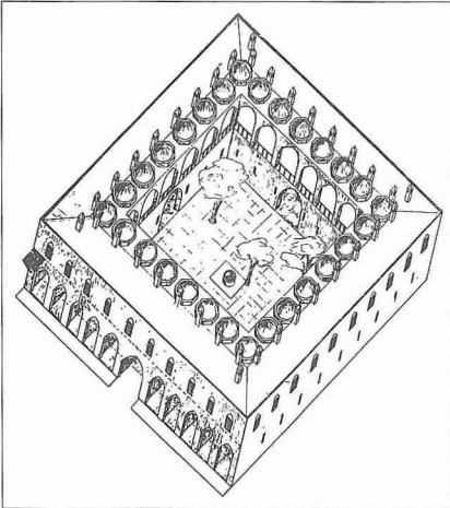
Elçi Hanı'nın tahmini olarak yapılmış restitüsyon denemesi (Ara Altun'un çizimi, S. Eyice'den)
