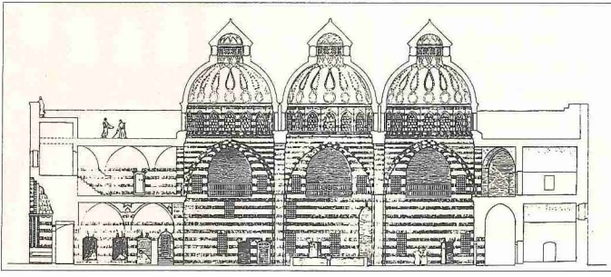
Esad Paşa Hanı'nın boyuna kesiti (Wulzinger-Watzinger, şekil 15)
