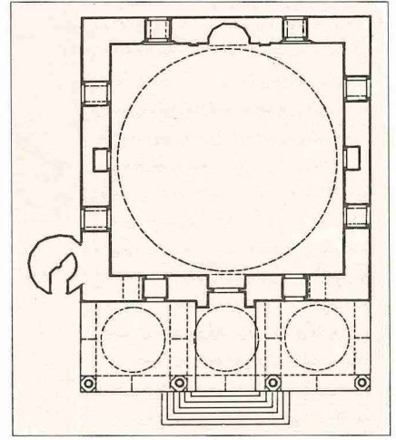
Fîruz Ağa Camii'nin planı
