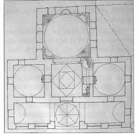
Firuz Bey Camii'nin planı
