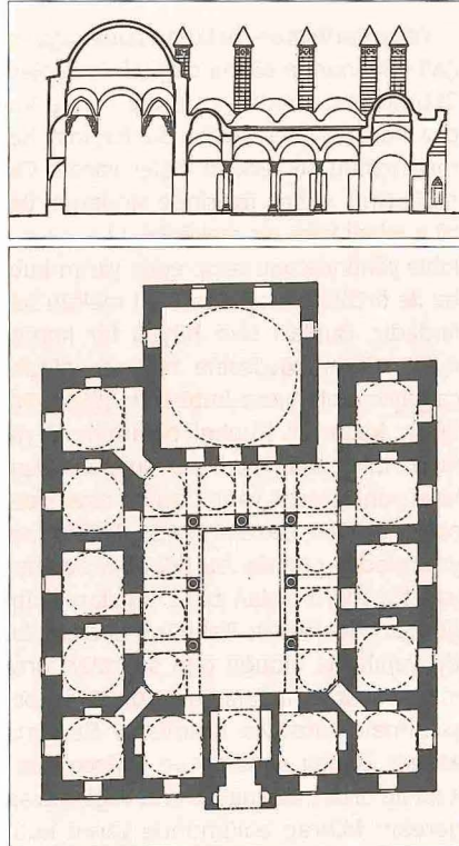
Gazi Hüseyin Bey Medresesi'nin planı ve kesiti
