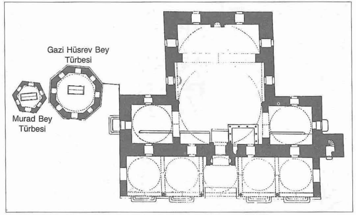
Gazi Hüsrev Bey Camii ve türbelerinin planı
