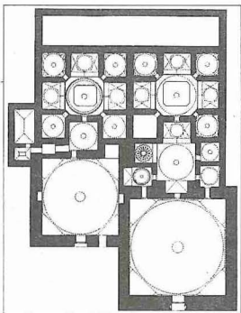
Gedik Paşa Hamamı'nın planı
