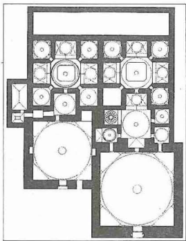
Gedik Paşa Hamamı'nın planı
