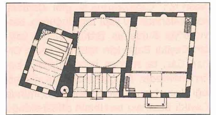
Geyikli Baba Camii ve Türbesi'nin planı
