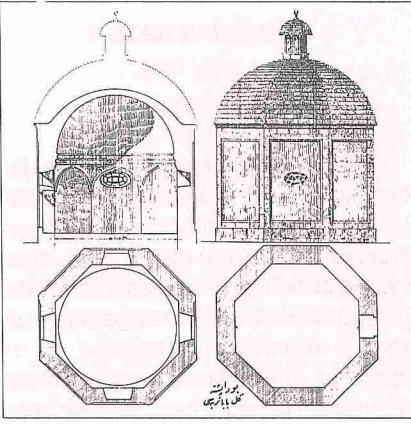
Gülbaba Türbesi'nin plan ve kesiti
