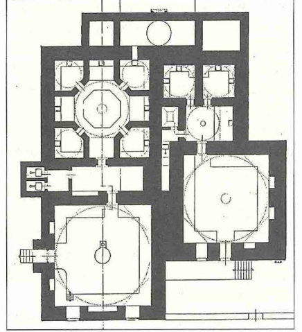
Hacı Hamza Hamamı'nın planı (Ülgen, I, rs. 85-A)
