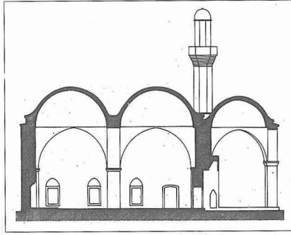
Dimetoka'daki Çelebi Sultan Mehmed Camii'nin kesiti
