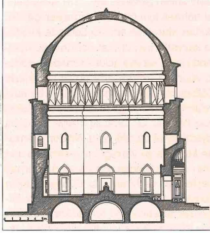
Yeşiltürbe'nin kesiti ile Hacı İvaz Paşa'nın Yeşilcami Külliyesi'ne vakif olarak inşa ettiği Geyve Hanı'nın planı
