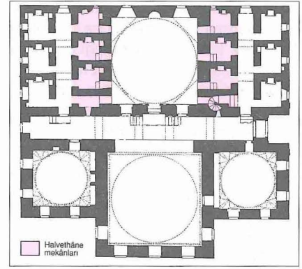
Amasya Yâkub Paşa Tekkesi'nin planı (Ayverdi, Osmanlı Mi'mârisi II , rs. 39)
