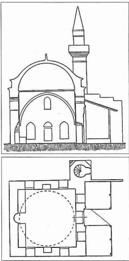
Rodos'ta Hamza Bey Camii'nin plan ve kesiti
