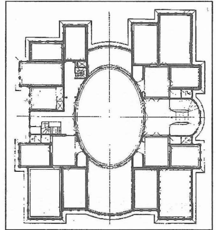
Hasib Paşa Yalısı Harem kısmının ikinci kat planı
