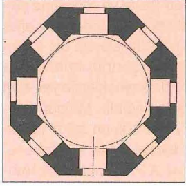
Hubbî Hatun Türbesi'nin planı
