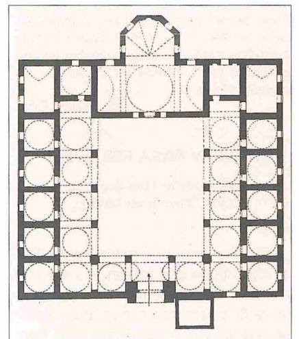
Hüsrev Paşa Camii - Medresesi'nin planı
