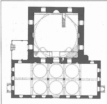
İshaklı Camii'nin planı
