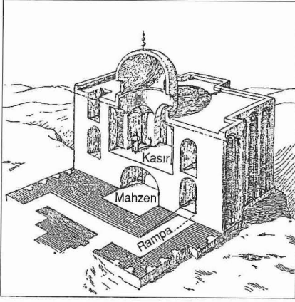
Kal'atü Benî Hammâd'ın başkulesinin (el-Menâr) kesiti (Marçais, Manuel d'art musulman , şekil 59)
