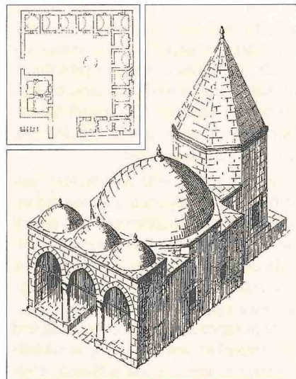
Karakurt Külliyesi'nde türbe ve caminin Yılmaz Önge tarafından çizilen restitüsyonu ile hankahın planı (Eyice, rs. 11)
