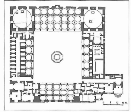
Ferec b. Berkuk Hankahı'nın planı
