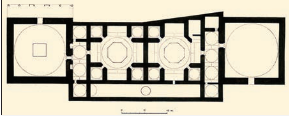
Kızlar Ağısı Hamamı'nın planı
