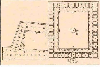
Koza Hanı'nın planı
