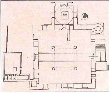
Mahmud Paşa Camii ve Türbesi'nin planı
