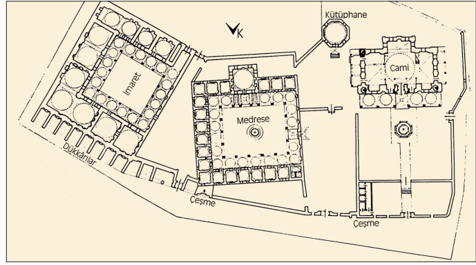
Manisa Murâdiye Külliyesi'nin planı
