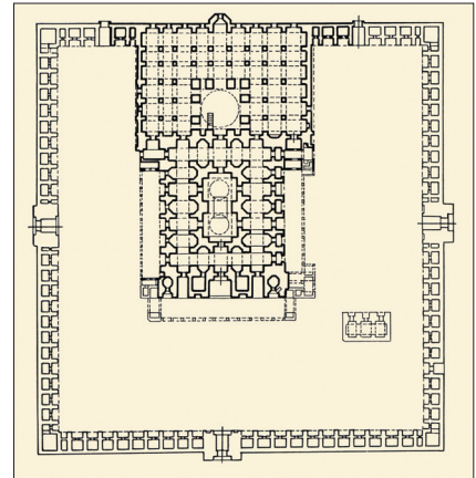
Mûsâ Kâzım Külliyesi'nin planı
