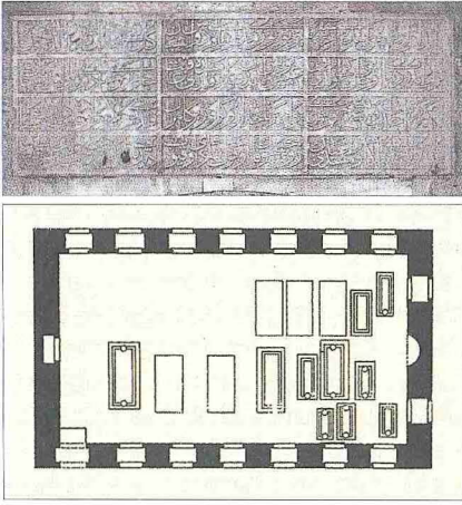
Pertev Paşa Türbesi'nin planı ve kitabesi
