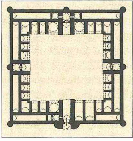
Serahs yolundaki Ribât-ı Mâhî'nin planı
