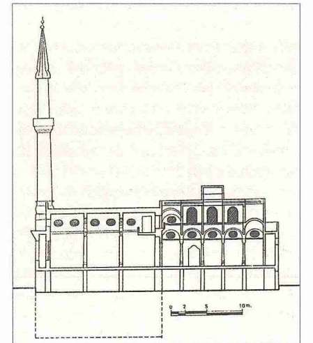
Silâhdar Süleyman Ağa Camii'nin güneydoğu cephesinin kesiti
