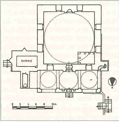
Süleyman Han Camii'nin planı
