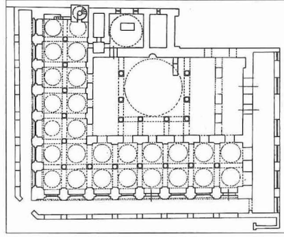
Âzamiye Camii ve Türbesi'nin planı
