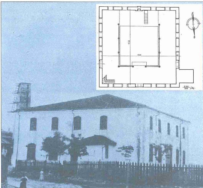
Aziziye Camii'nin 1880 yılına ait bir resmi - Dobruca / Romanya (İÜ Ktp., Albüm, nr. 91.233) ve planı (Ayverdi'den)
