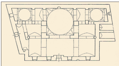
Timurtaş Paşa Camii'nin planı
