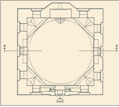
Urfa Mevlevihânesi semâhânesinin planı ile kesiti (Vakıflar Genel Müdürlüğü Arşivi)
