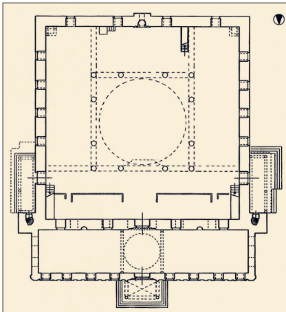
Çorum Ulu Camii'nin planı
