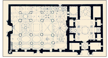
Divriği Ulucamii ve Şifâhânesi'nin planı
