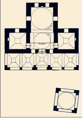
Yâkub Celebi Zâviyesi ve Türbesi'nin planı
