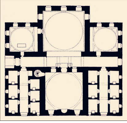
Yâkub Paşa Tekkesi'nin planı
