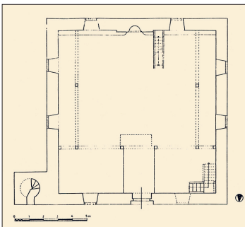
Artvin Zeytinlik Camii'nin planı ve güney cephesi
