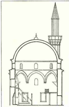
Bayraklı Cami'nin plan ve kesiti (Ayverdi, III, resim 876-877)
