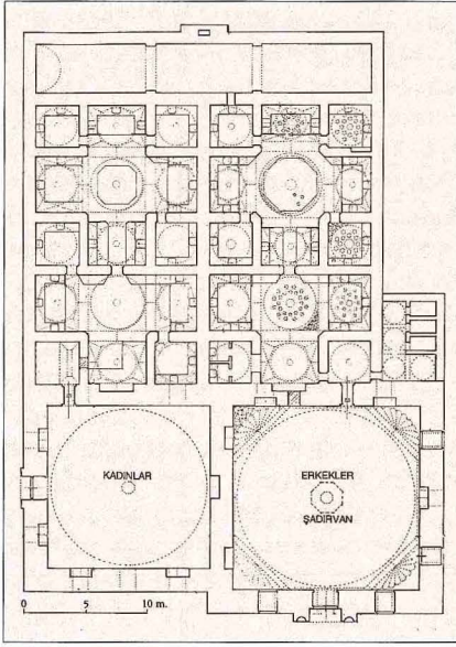
Beyazıt Hamamı'nın planı (İ. Aydın Yüksel'den)
