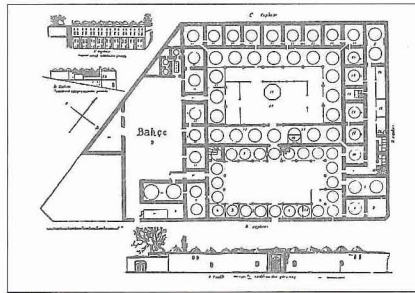
Süleymaniye Dârüşşifâsı ve Tıp Medresesi ile dârüşşifânın planı - İstanbul
