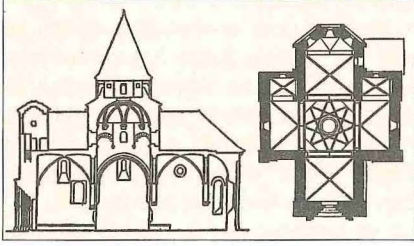
Turan Melik Dârüşşifâsı'na benzeyen Hospital de Saint Blaise'in plan ve kubbe konstrüksiyonu
