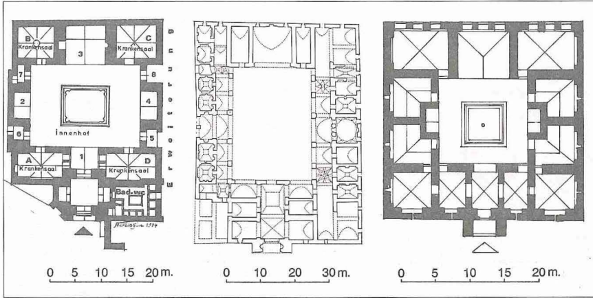
Şam'daki Nüreddin Bimaristanı'nın planı (A. Terzioğlu'ndan), Keykâvus Dârüşşifâsı'nın planı ve Dimâşk'ta 1248'de tesis edilen Kaymerî Bimaristanı'nın planı
