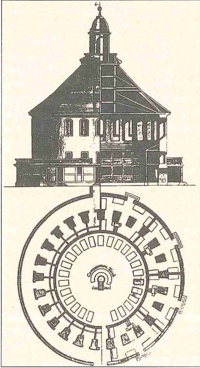
L. Ch. Sturm tarafından 1920'de merkezî şekilde planlanmış hastahane projesi
