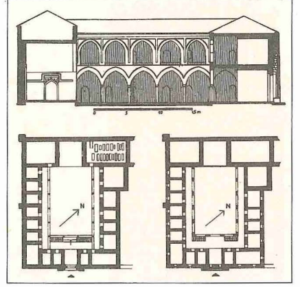
Gökmedrese'nin plan ve kesiti (A. Gabriel'den)
