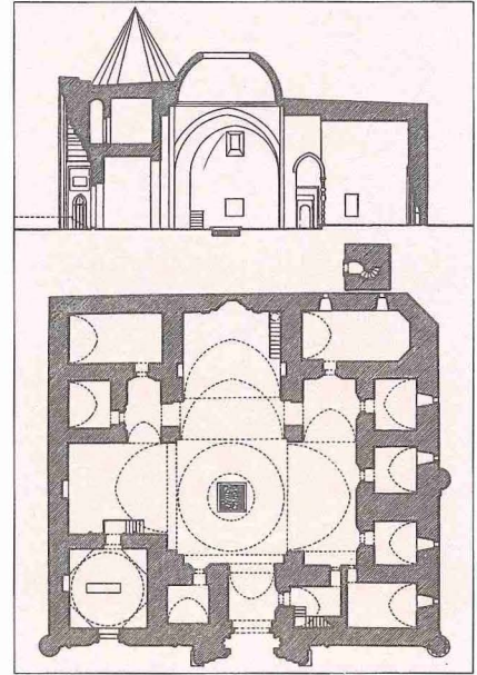
Caca Bey Medresesi'nin planı ile boyuna kesiti (A. Kuran, Anadolu Medreseleri , I, şekil 25-26)
