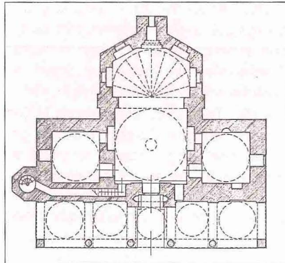
Tîre Yahşi Bey (Yeşilce İmareti) Camii'nin planı
