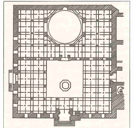
Manisa Ulucamii'nin planı
