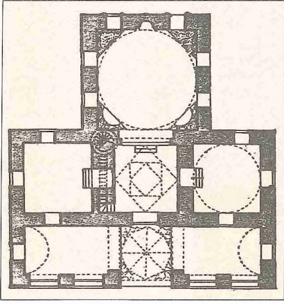
Menteşeoğulları'na ait Firuz Bey Camii ve planı - Milas / Muğla
