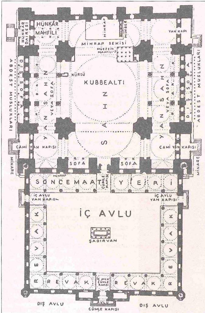
Klasik Osmanlı devri camilerinin kısmı ile düzenlemesi gösteren sematik plan
