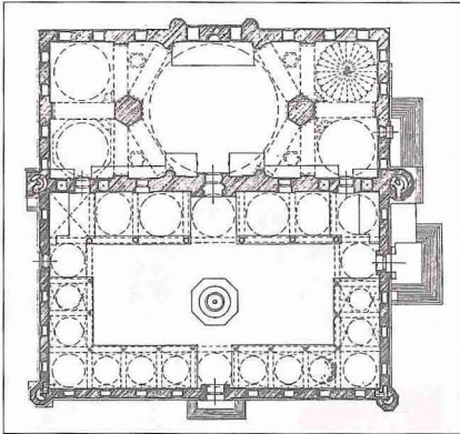
Edirne'de Üç Şerefeli Cami ve planı
