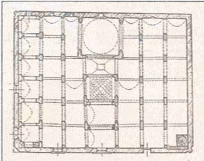
Erzurum Ulucamii'nin planı
