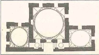
Bursa Yenişehir'de Postinpüş Baba Zâviye-Camii ve planı
