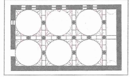
Antalya Yivli Minare Camii'nin planı
