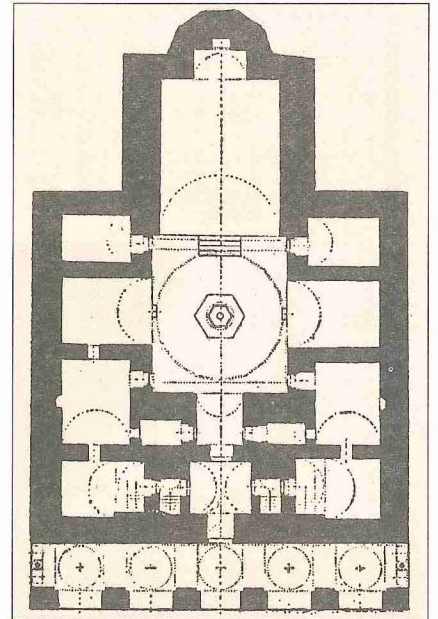
Bursa Hüdâvendigâr Camii'nin alt kat planı
