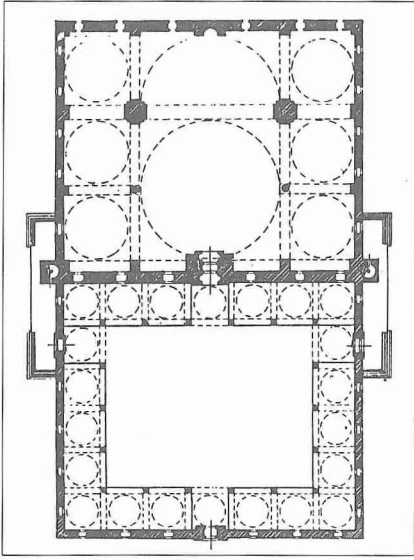
İstanbul'da eski Fâtih Camii'nin planı
