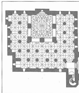
Van Ulucamii'nin planı ve Anadolu'nun pâyeli tipteki ilk camilerinden biri olan Ani Camii - Ocaklı köyü / Kars
