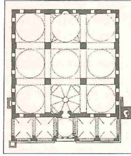
Edirne'de Eski Camii ve planı
