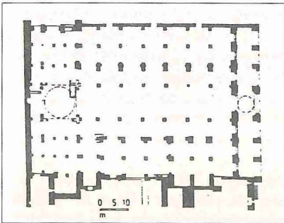
Mescid-i Aksâ ve planı - Kudüs
