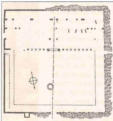
Suriye'deki Rakka Ulucamii'nin planı ile Harran Ulucamii'nin planı (K. A. C. Creswell, Early Muslim Architecture, s. 151, şekil 29)
