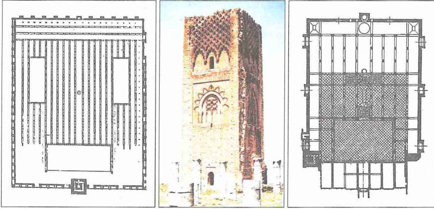
Hassan Camii'nin planı ve dört köşeli minaresi ile Tâzâ Camii'nin planı - Fas
