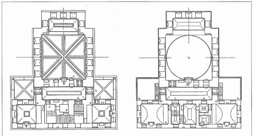
Dâvud Paşa Sarayı'nın üst ve alt kat planları (Eldem, rs. 150, 151)
