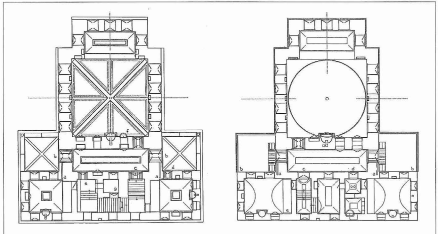
Dâvud Paşa Sarayı'nın üst ve alt kat planları (Eldem, rs. 150, 151)
