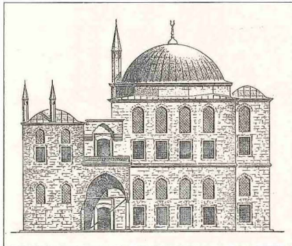
Dâvud Paşa Sarayı'nın güneybatı cephesinin kesiti ile çizimi (Eldem, rs. 152, 153)
