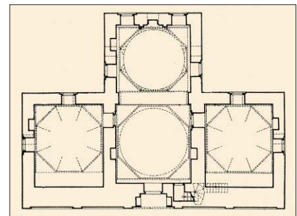
Koca Mehmed Paşa Camii'nin planı
